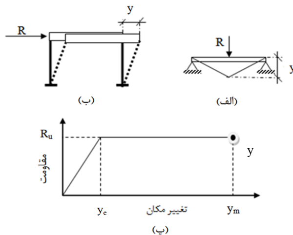
شکل ۳-۵-۲۱- سازه یک‌درجه آزادی ارتجاعی - خمیری
