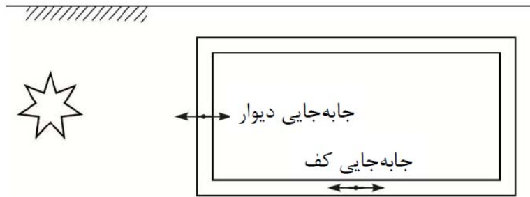
شکل ۳-۲۱-۱۳- حرکات افقی دیوار و کف
