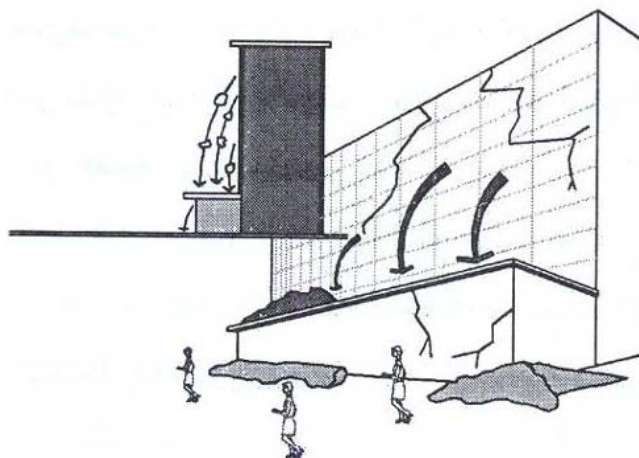
شکل ۲-۲۱-۴- شکل‌های مناسب نمای ساختمان برای کاهش ریزش آوار به محیط
